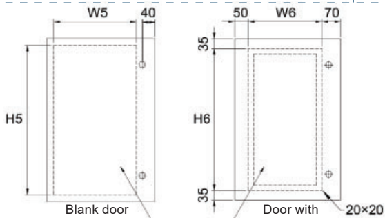
Door
